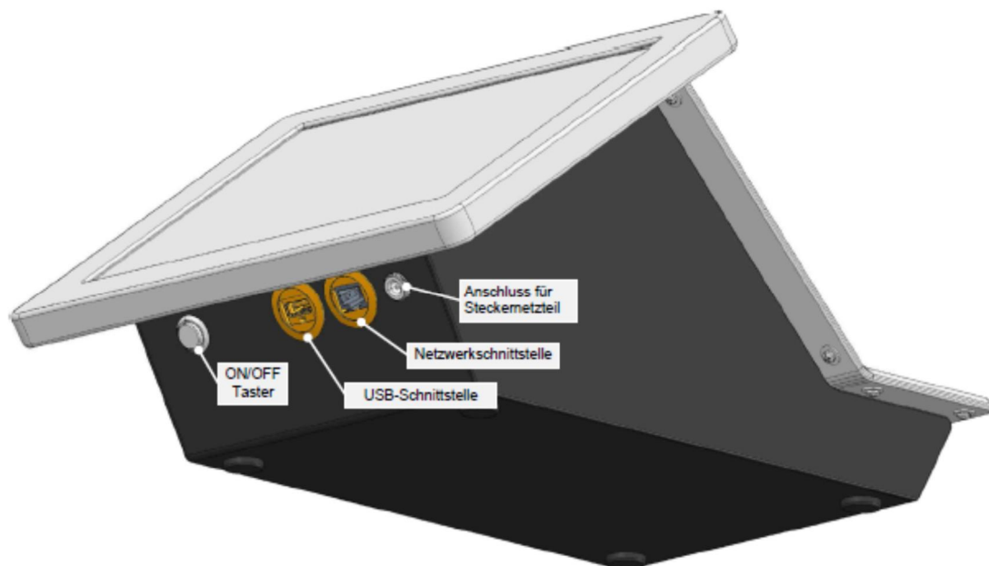
Abbildung 1 - Anschlüsse Bedienerseite
